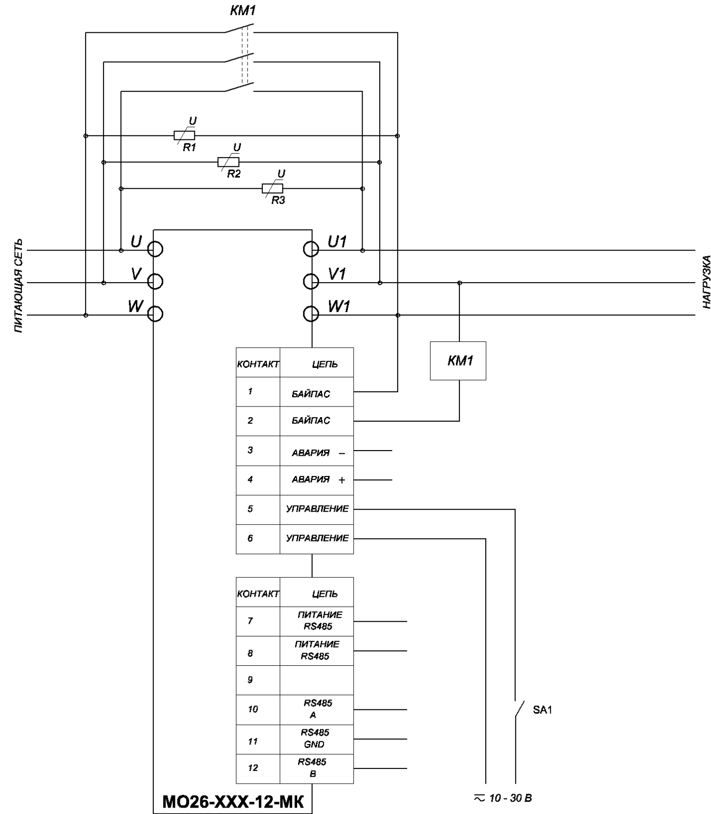
Рисунок 4.1 – Схема подключения МО26-XXX-12-МК
