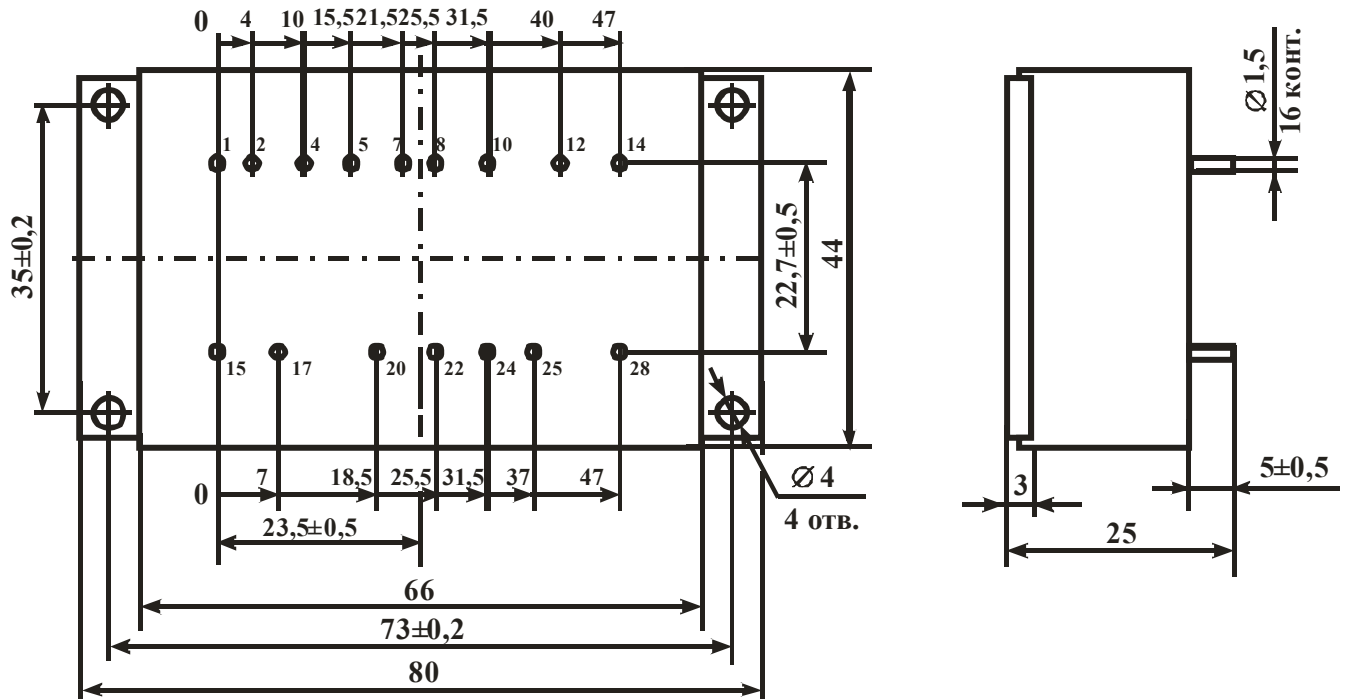
Рисунок 1 – Габаритный чертеж модуля: M13МСГ-30-6(12)
