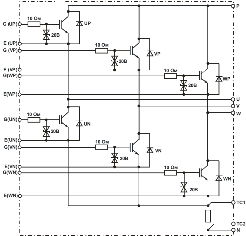
Рисунок 2 – Функциональная схема модуля
