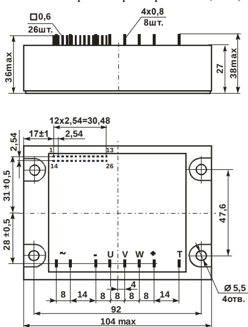
Рисунок 8.5 – Габаритные размеры М31-5,10-1,2,6А1*
