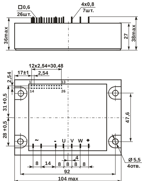
Рисунок 8.3 – Габаритные размеры МЗ1-5,10-1,2,6АЗ*
