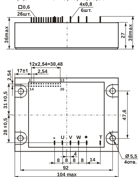
Рисунок 8.4 – Габаритные размеры МЗ1-5,10-1,2,6А2*
