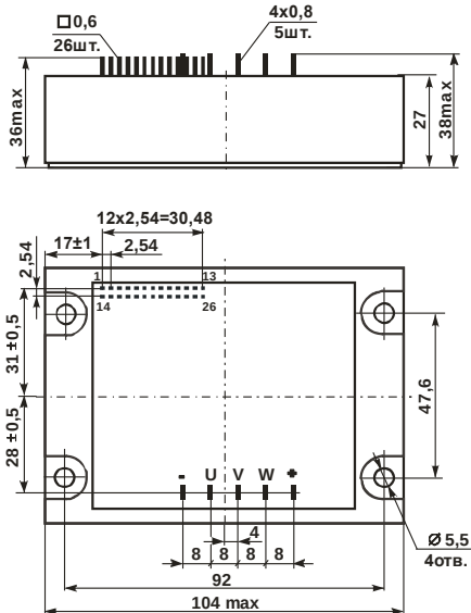
Рисунок 8.1 – Габаритные размеры МЗ1-5,10-1,2,6А4*
