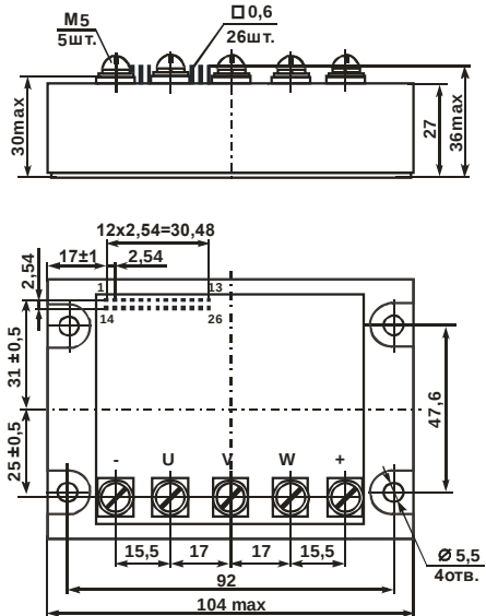
Рисунок 8.2 – Габаритные размеры М31-20,30,50,70,100-1,2,6А4 и М31-5,10,20,30,50-12А4*
