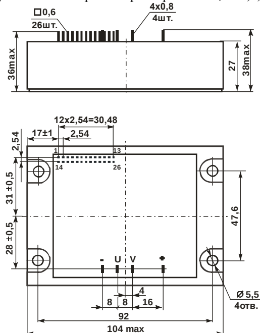
Рисунок 8.6 – Габаритные размеры МЗ1-5,10-1,2,6Б4*
