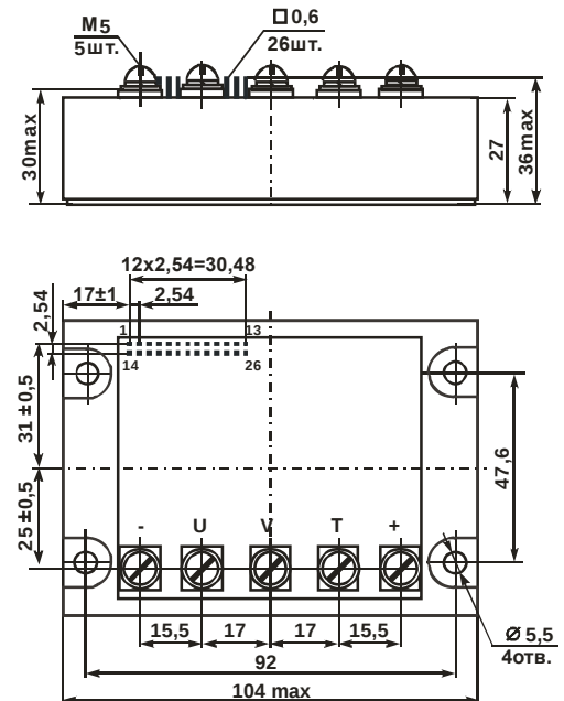
Рисунок 8.10 – Габаритные размеры М31-20,30,50,70,100-1,2,6Б2 и М31-5,10,20,30,50-12Б2*
