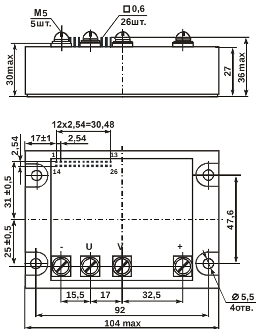
Рисунок 8.7 – Габаритные размеры М31-20,30,50,70,100-1,2,6Б4 и М31-5,10,20,30,50-12Б4*
