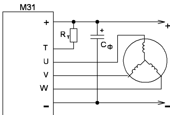
Рисунок 6.1 – Схема подключения M31 с типом силовой сборки «4»
