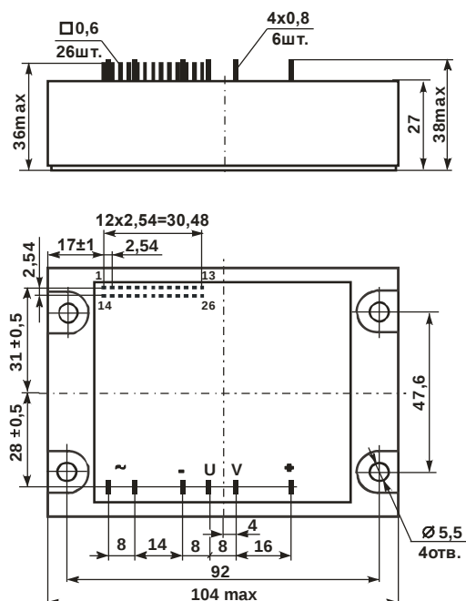
Рисунок 8.8 – Габаритные размеры М31-5,10-1,2,6Б3*
