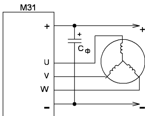
Рисунок 6.1 – Схема подключения M31 с типом силовой сборки «4»
