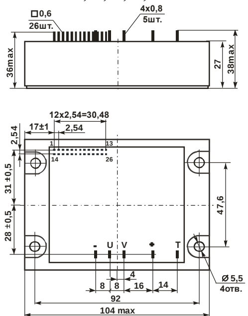
Рисунок 8.9 – Габаритные размеры М31-5,10-1,2,6Б2*
