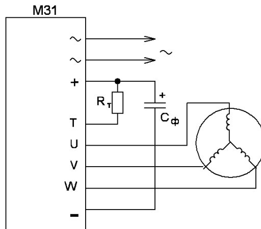
Рисунок 6.4 – Схема подключения M31 с типом силовой сборки «1»
