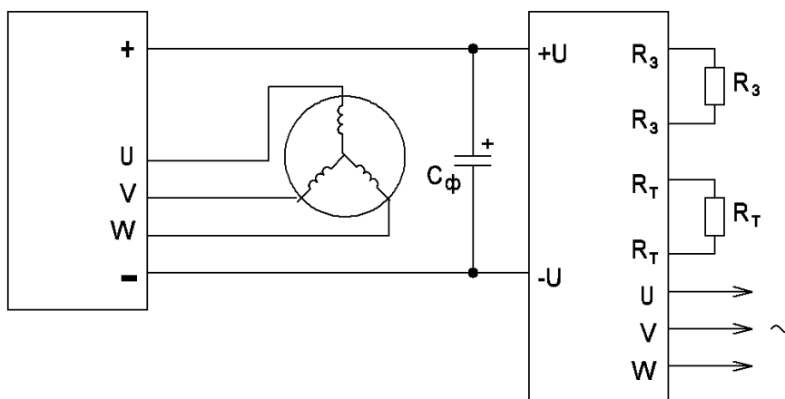
Рисунок 6.5 – Схема подключения M31 с типом силовой сборки «4» в составе с МККН
