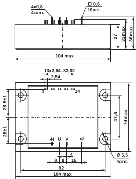
Рисунок 1 – Габаритный чертеж модулей: М13Б-10-2
