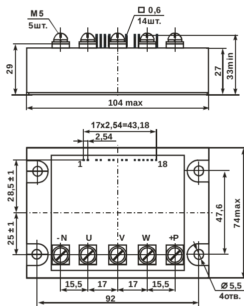
Рисунок 2 – Габаритный чертеж модулей: М13А-30-1, М13А-50-1, М13А-90-1
