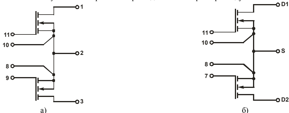
а) Рисунок 2 – Электрическая схема внутренних соединений модуля
