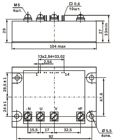
Рисунок 2 – Габаритный чертеж модулей: М13Б-30-2, М13Б-50-2, М13Б-90-2
