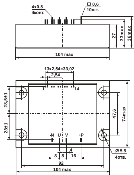
Рисунок 1 – Габаритный чертеж модулей: M13Б-10-1
