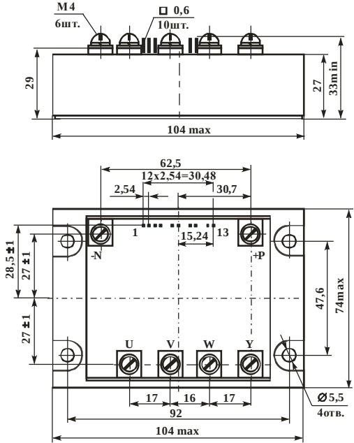
Рисунок 2 – Габаритный чертеж модуля M13B-30-1; M13B-50-1; M13B-90-1
