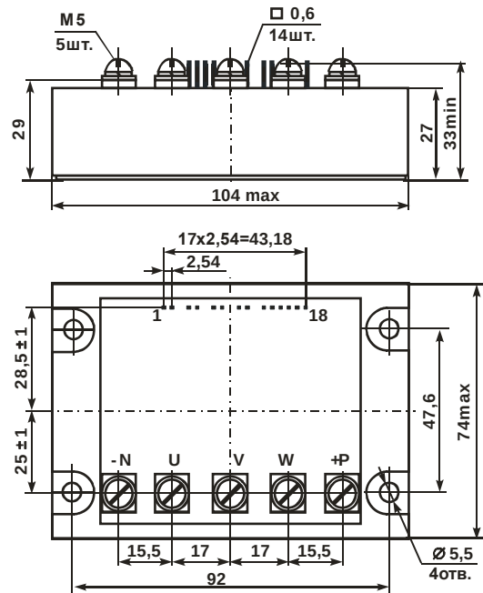
Рисунок 2 – Габаритный чертеж модулей: M13A-30-2, M13-50-2, M13-90-2
