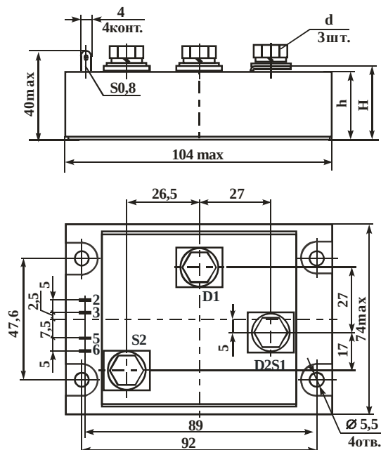
Рисунок 1 – Габаритные и присоединительные размеры модуля
