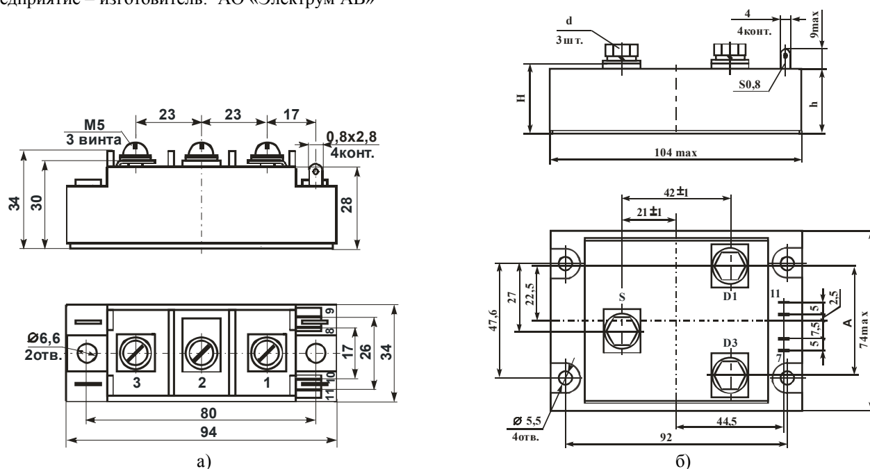
а) Рисунок 1 – Габаритные и присоединительные размеры модуля
