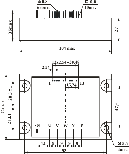
Рисунок 1 – Габаритный чертеж модуля M13B-10-1
