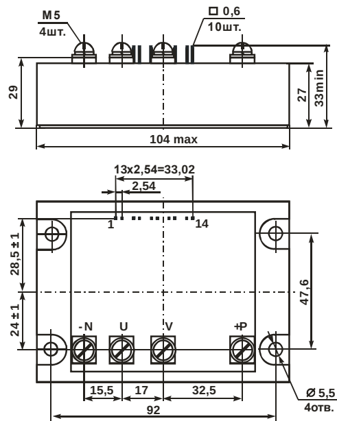
Рисунок 2 – Габаритный чертеж модулей: M13Б-30-1, M13Б-50-1, M13Б-90-1
