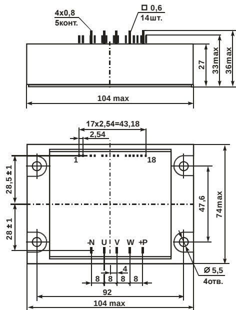
Рисунок 1 – Габаритный чертеж модулей: М13А-10-1
