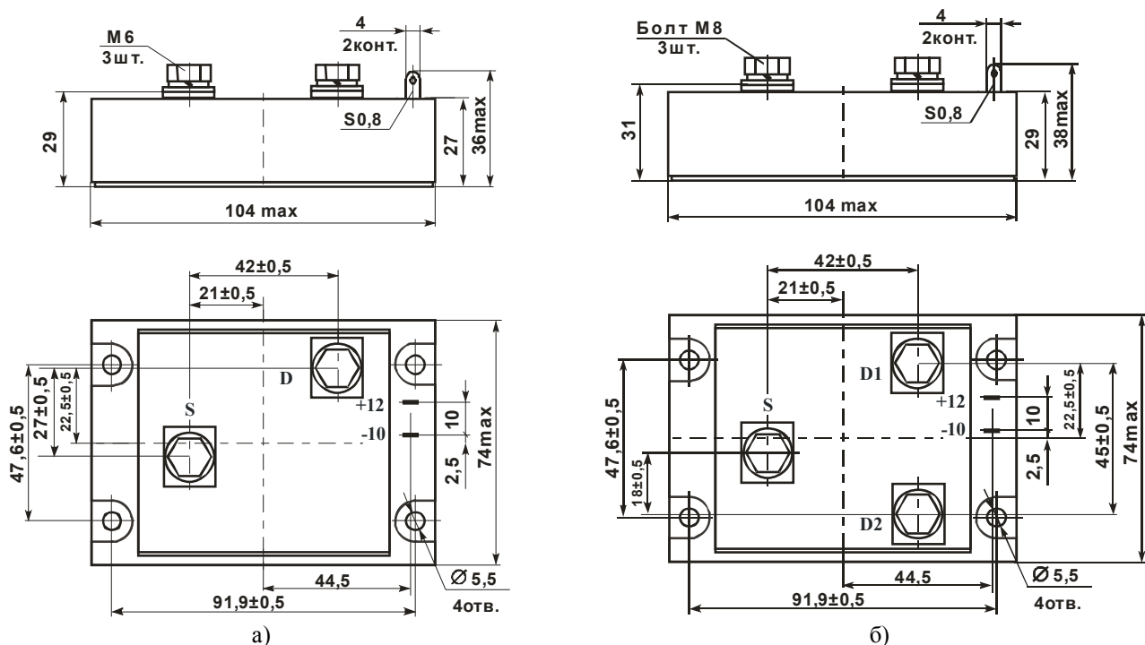
Рисунок 1 – Габаритные и присоединительные размеры модуля
