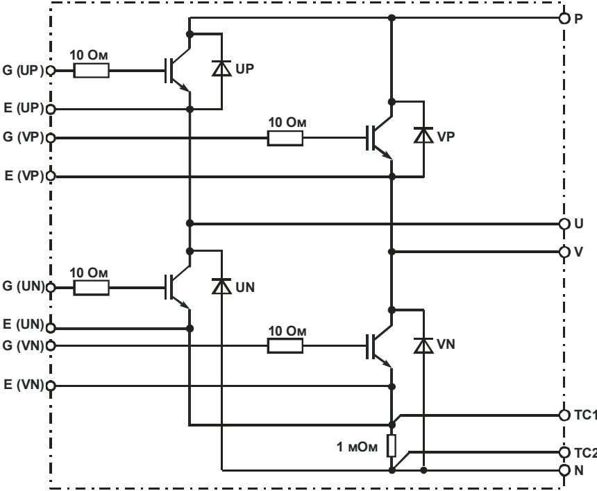
Рисунок 3 – Функциональная схема модуля
