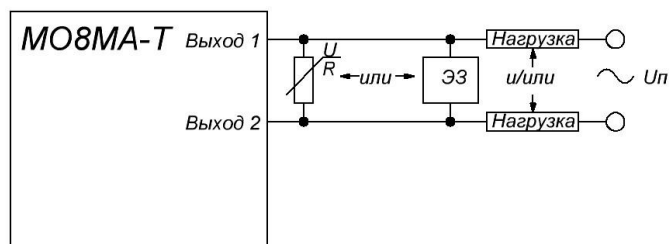
а) Схема подключения модуля с встроенным шунтом
