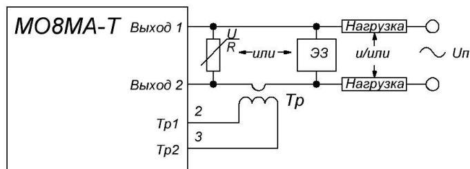
б) Схема подключения модуля с внешним токоизмерительным трансформатором
