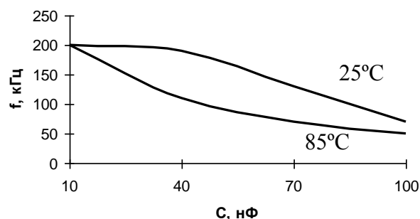
Рисунок 6 – График области безопасной работы драйвера для емкостей затвора от 10 до 100 нФ при температуре окружающей среды 25^{\circ}\text{C} и 85^{\circ}\text{C}
